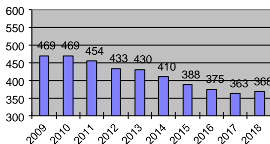
Spezifischer Energieverbrauch in kWh/t Papier
