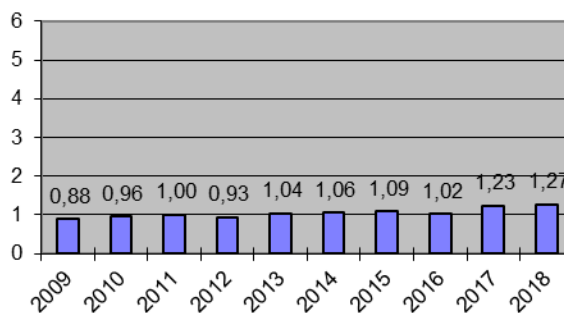
Spezifischer Abwasseranfall in l/kg Papier
