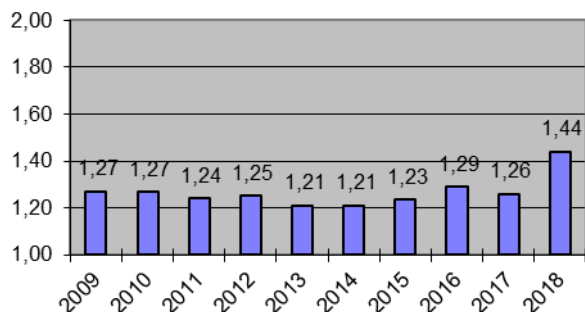
Spezifischer Dampfverbrauch in tD/t Papier
