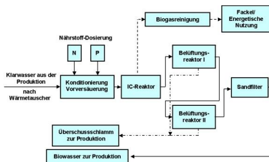
Abb.: Verfahrensschema der Kreislaufwasserbehandlungsanlage (KWB)
